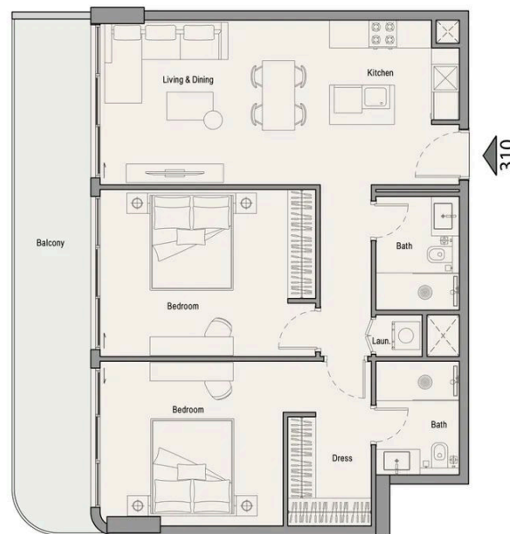
UNIT 310 - 2 BEDROOM
